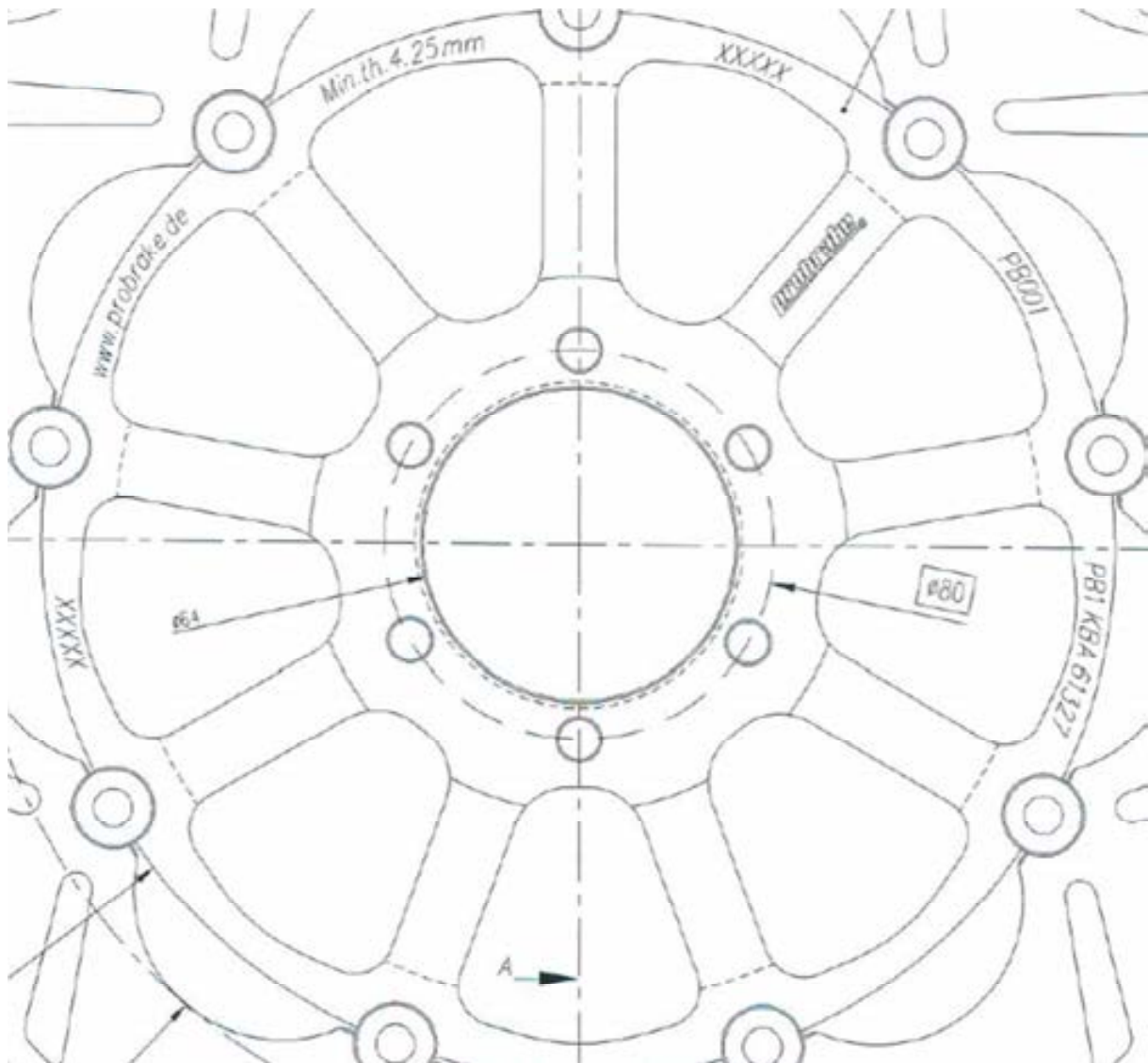
Kennzeichnungen der Bremsscheibe
